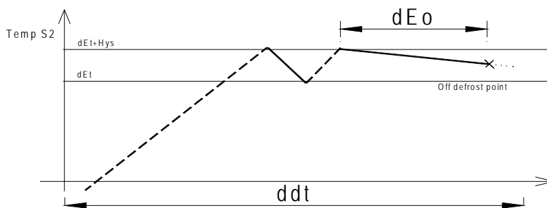
Fig1: Fonctionnement de l'optimisation du dégivrage.
